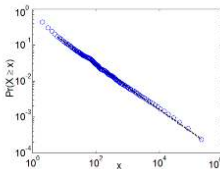
شکل ۱: نمودار تابع توزیع تجمعی تعداد تکرار عبارت‌ها در پرس و جوهای خام
