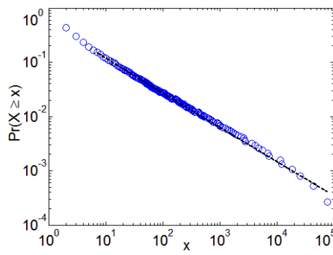
نمودار ۳- تابع توزیع تجمعی تعداد تکرار عبارت‌ها در پرس‌وجوهای بازآرایی شده
